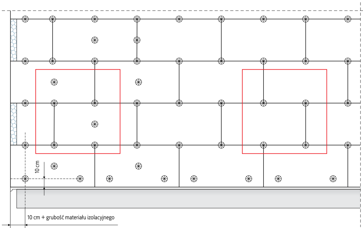
Rys. 5 Przykładowe rozmieszczenie łączników mechanicznych mocujących płyty styropianowe na wysokości do 8 m nad poziomem terenu.
