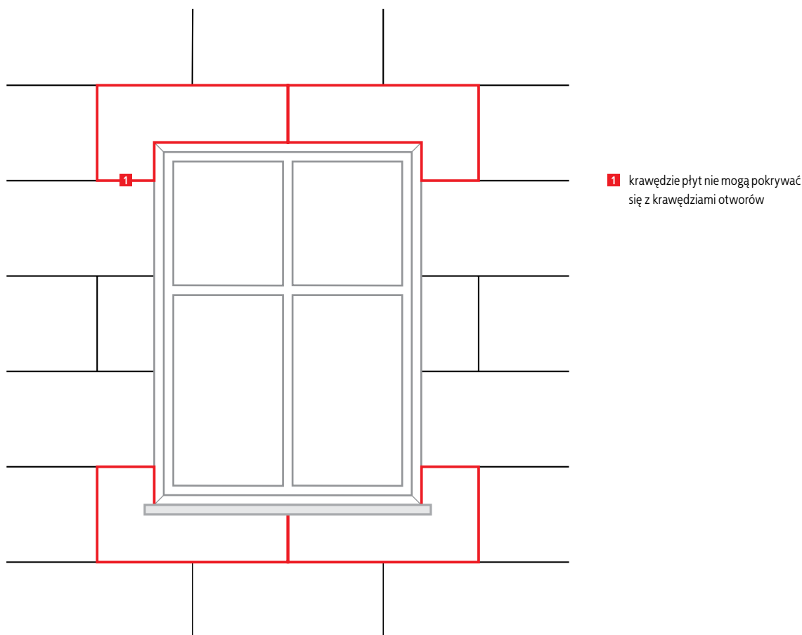
Rys. 4 Montaż płyt styropianowych w obrębie otworów elewacji.
