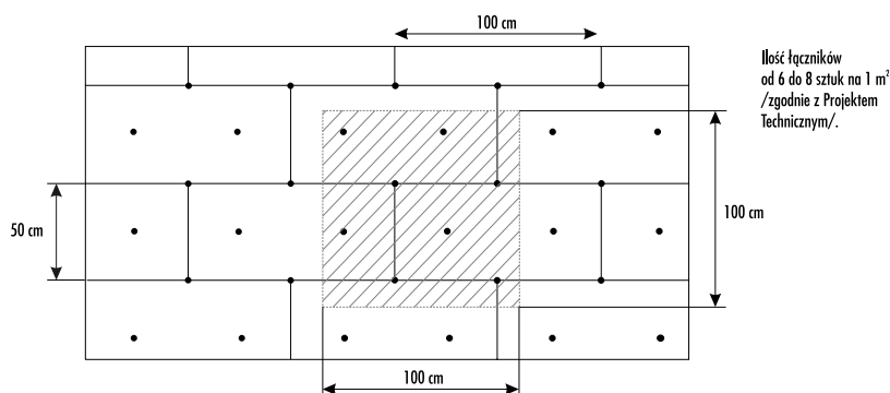
Rys. 13 Przykładowe rozmieszczenie łączników mechanicznych na powierzchni płyt z fasadowej wełny mineralnej
