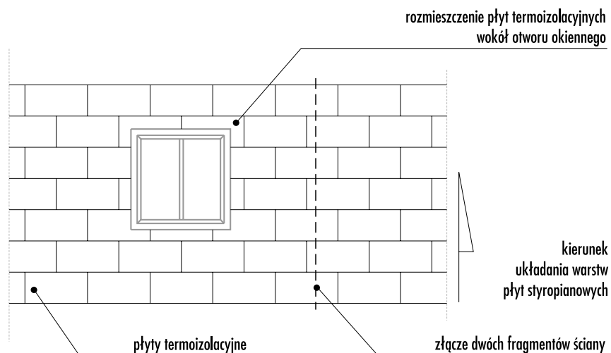
Rys. 5/ Schemat rozmieszczenia płyt termoizolacyjnych na powierzchni ściany
