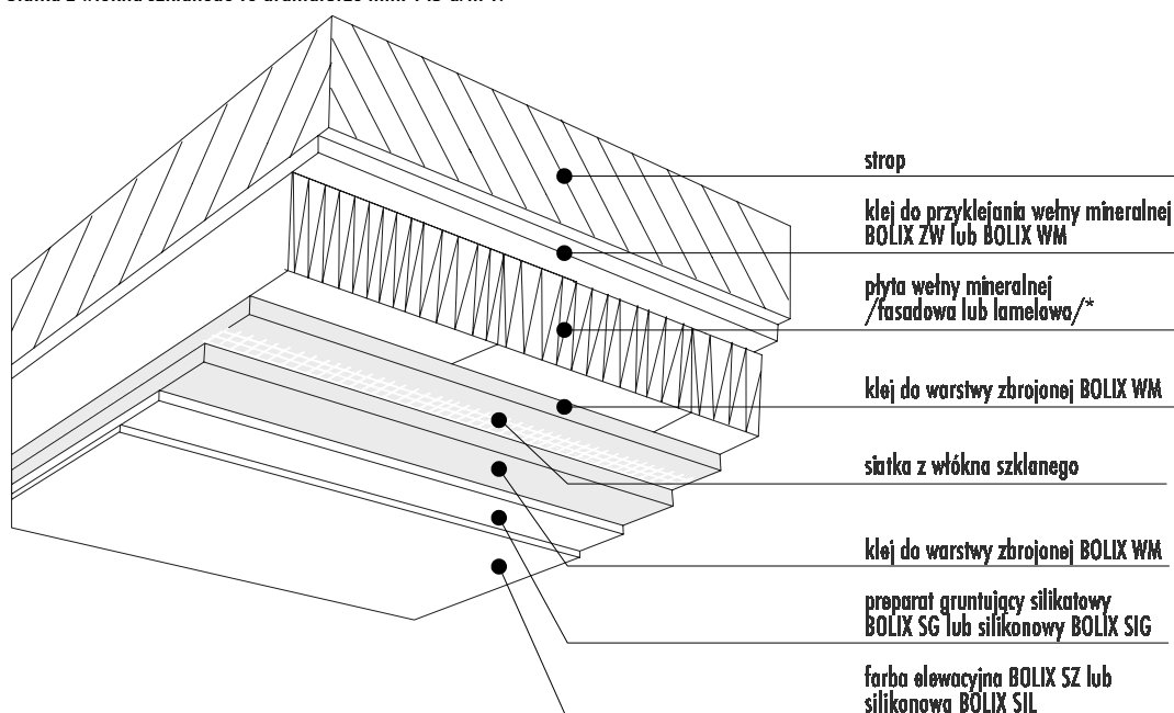
Rys. 28/ Elementy systemu ociepleń BOLIX M1-G
