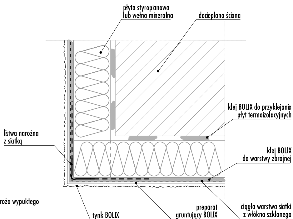
- NAROŻE WYPUKŁE (przekrój poziomy)
