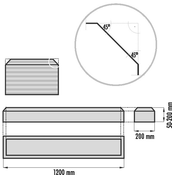
Rys. 30/ Rysunek schematyczny sfazowanej wełny stosowanej w systemie BOLIX IZO-Strop
