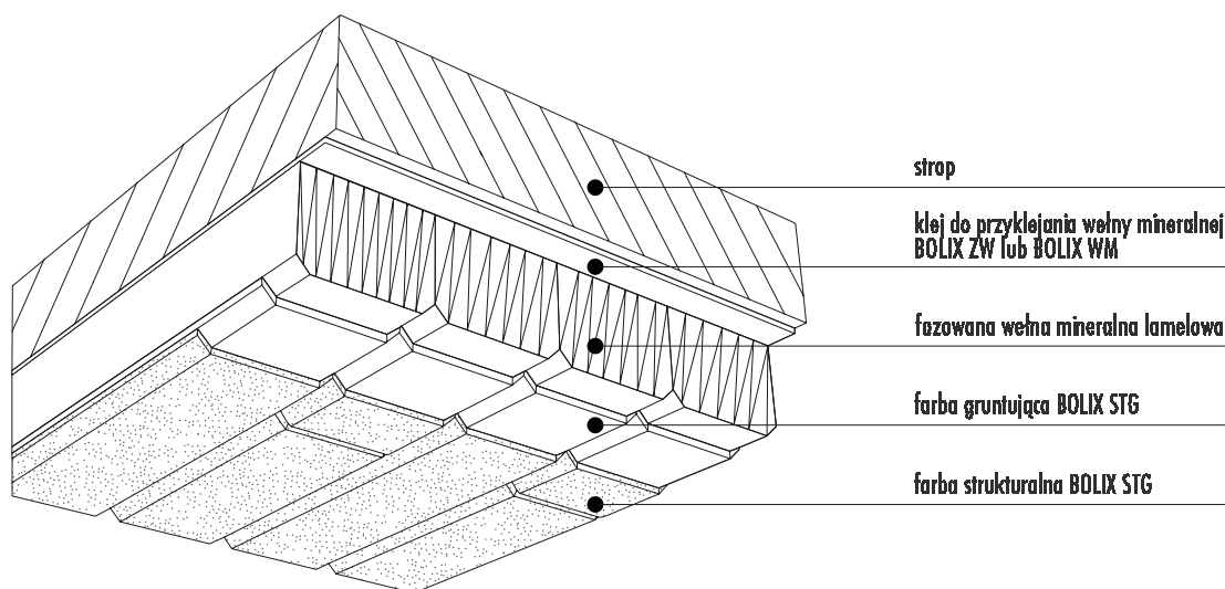
Rys. 29/ Elementy systemu ociepleń BOLIX IZO-Strop
