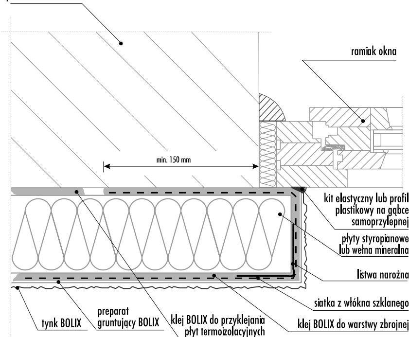
Rys. 21/ Detal docieplenia przegrody przy oknach licujących ze ścianą zewnętrzną
