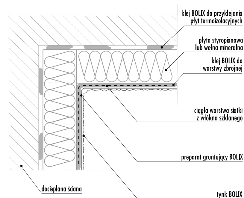
- NAROŻE WKŁĘSŁE (przekrój poziomy)
