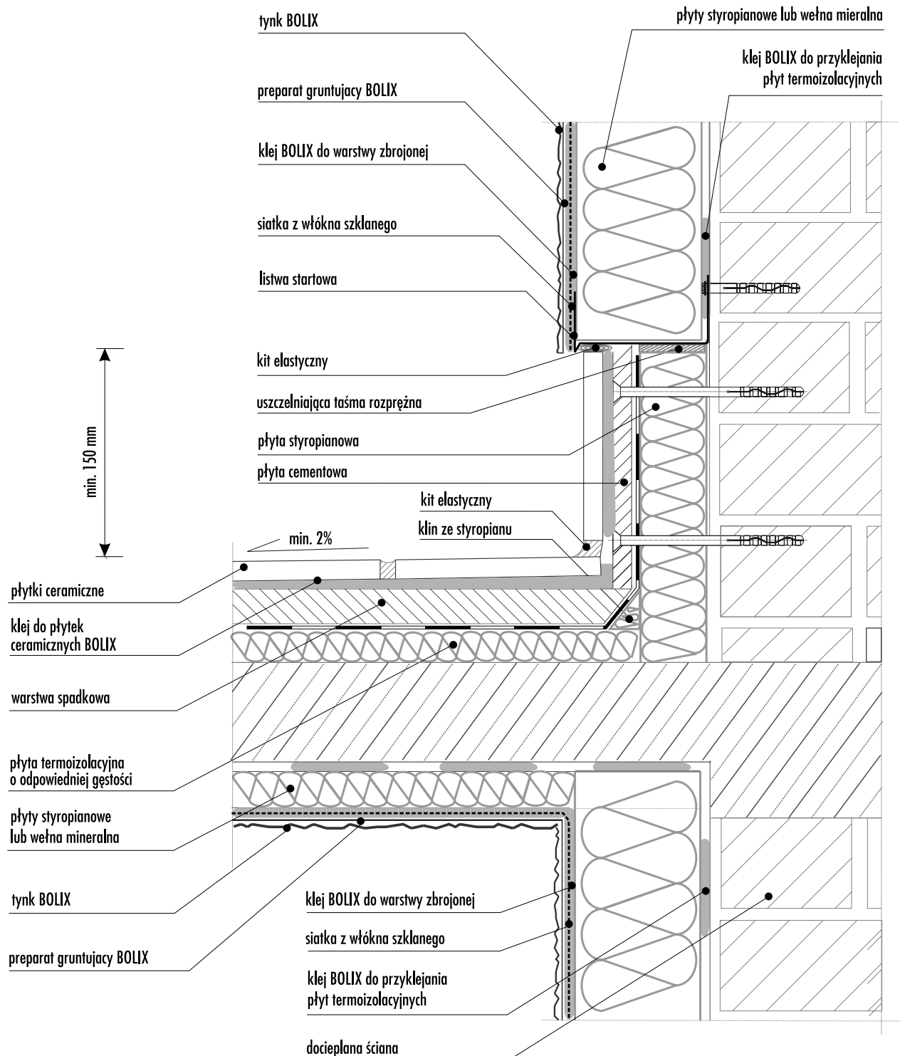
Rys. 27/ Detal docieplenia ścian przy połączeniu z balkonem lub loggią
