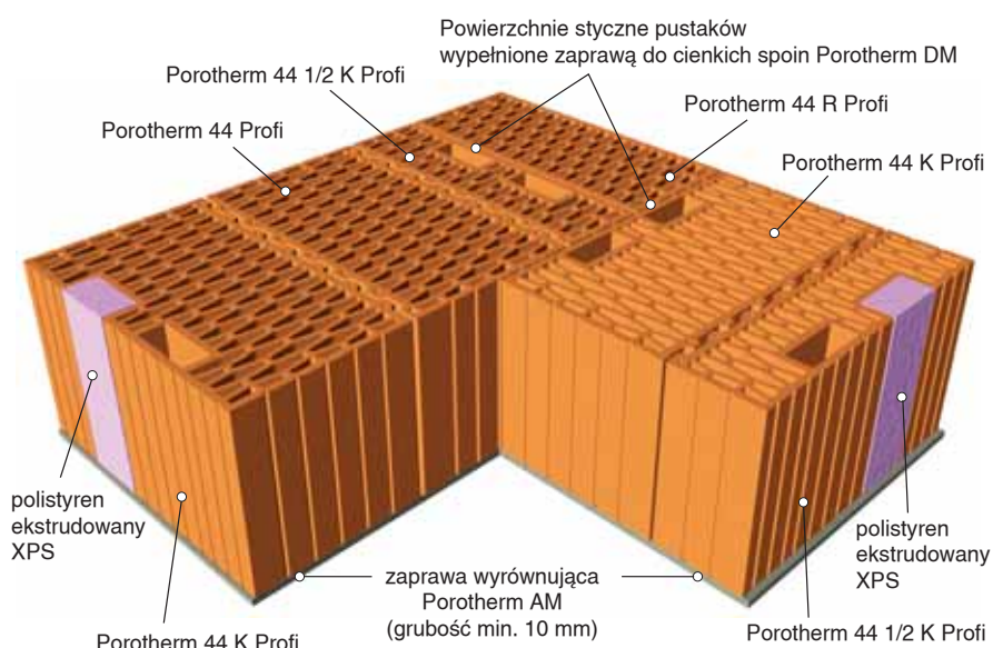
rys. 18 Schemat prawidłowo wykonanego narożnika
